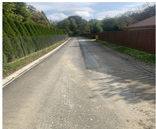
Przebudowa drogi gminnej - nawierzchnia asfaltowa dz. nr 699 – ul. Działowa w Błazowej.
